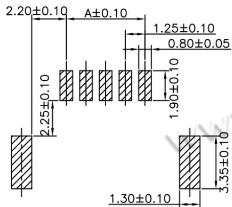
P.C.B. LAYOUT
